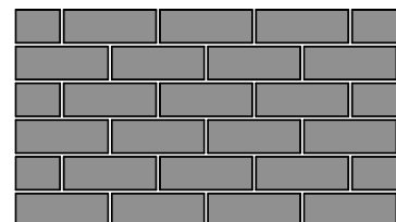
Halbversetzter Läuferverband
