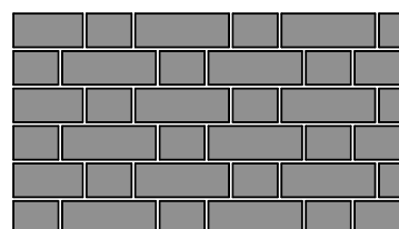
Flämischer Verband
