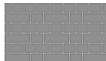
Holländischer Verband
