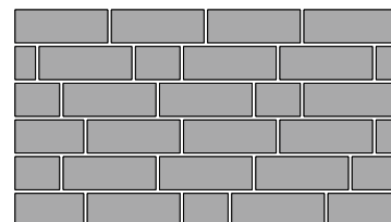
Wilder Verband
