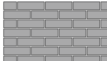
NF-Format 240/115/71 mm
