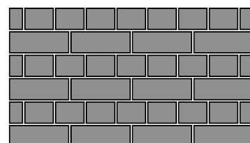
Kreuzverband
